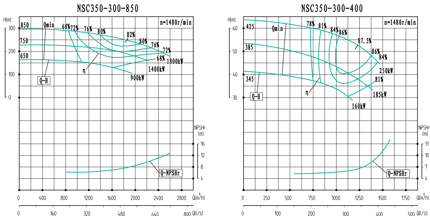
性能曲线图
