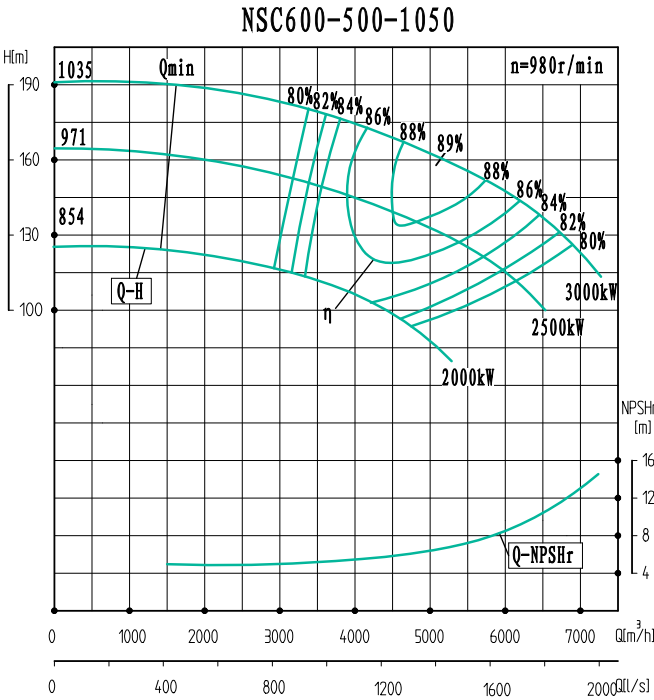
性能曲线图
