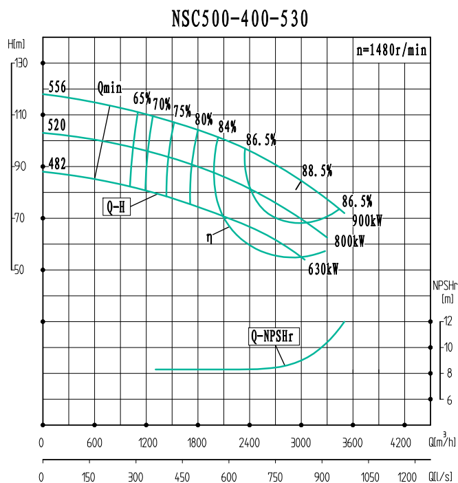
性能曲线图
