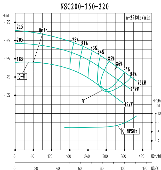
性能曲线图
