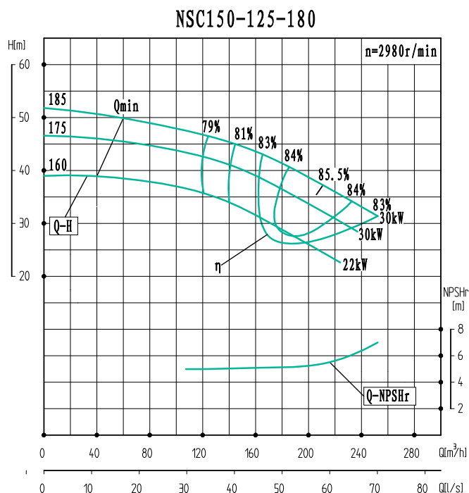
性能曲线图
