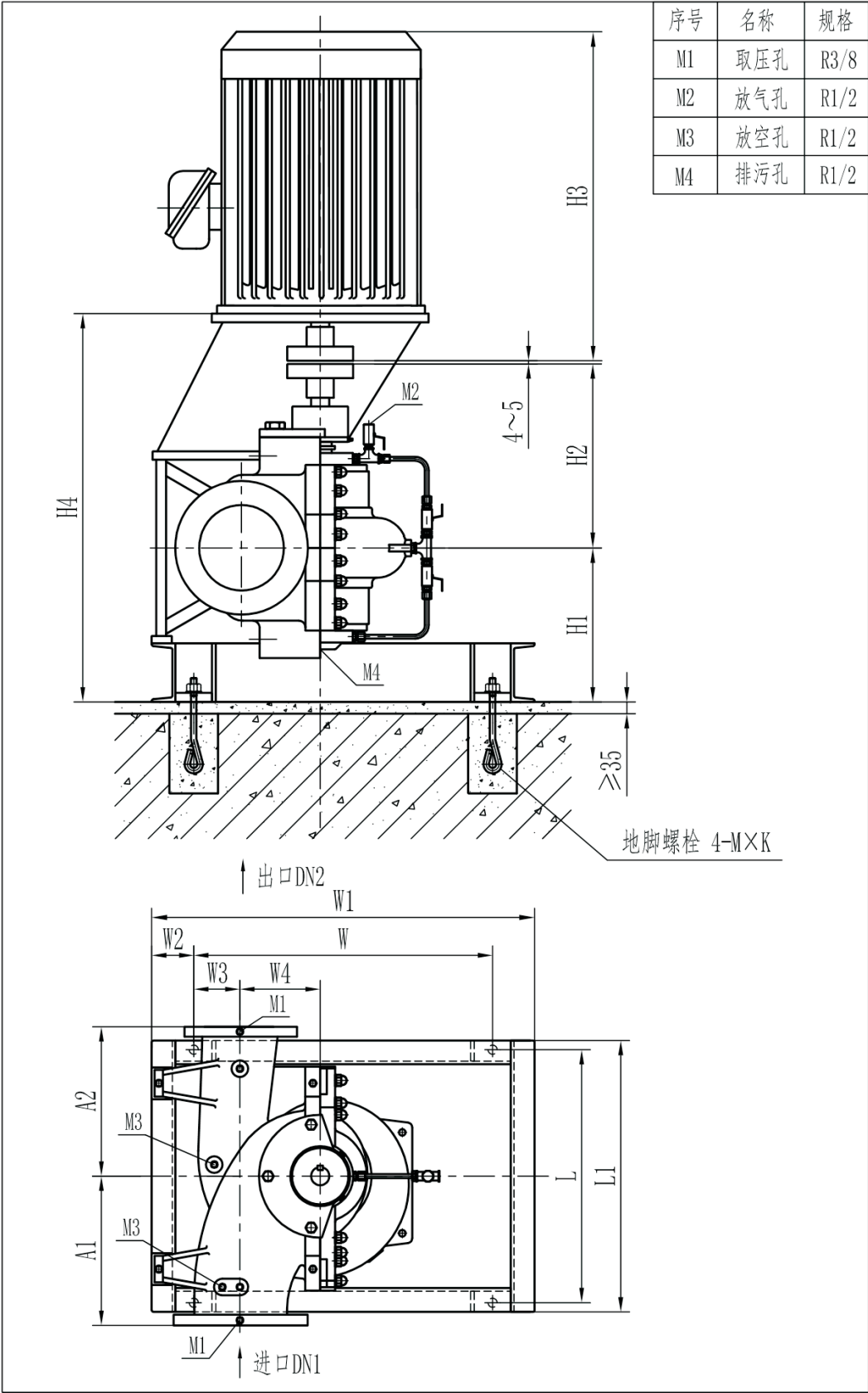
立式安装泵机组外形尺寸
