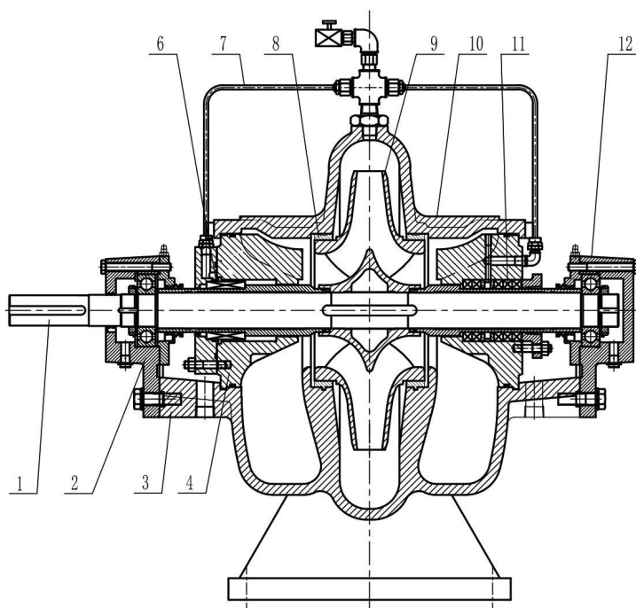
▲A型结构图
