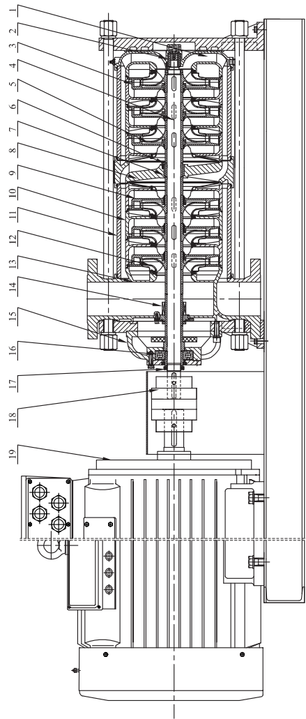
截面图 VMHP130-6, 210-6
