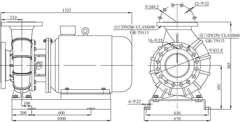
安装图CH250-200-315/75
