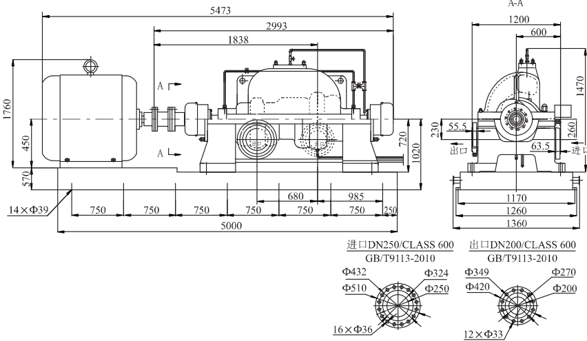
安装图VMHP520-5
