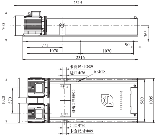
安装图VMHP42-15×2
