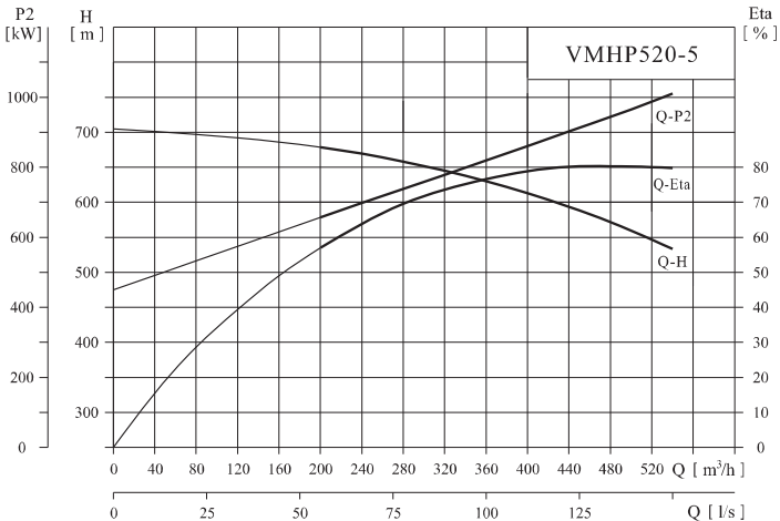
性能表VMHP520-5
