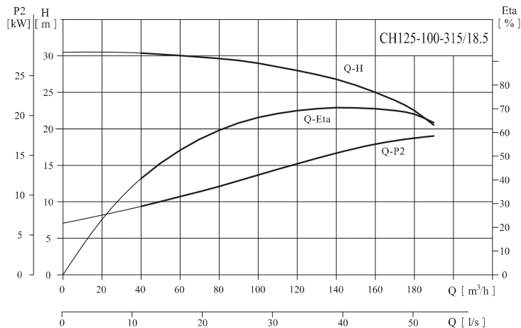
性能表CH125-100-315/18.5
