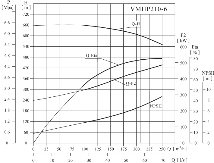
性能表VMHP210-6
