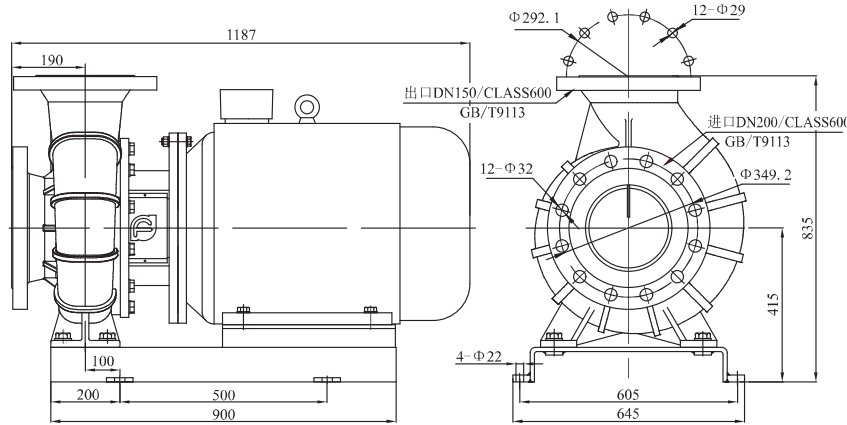
安装图CH200-150-315/45
