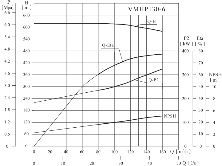
性能表VMHP130-6
