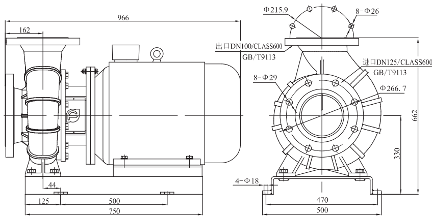
安装图CH125-100-315/18.5
