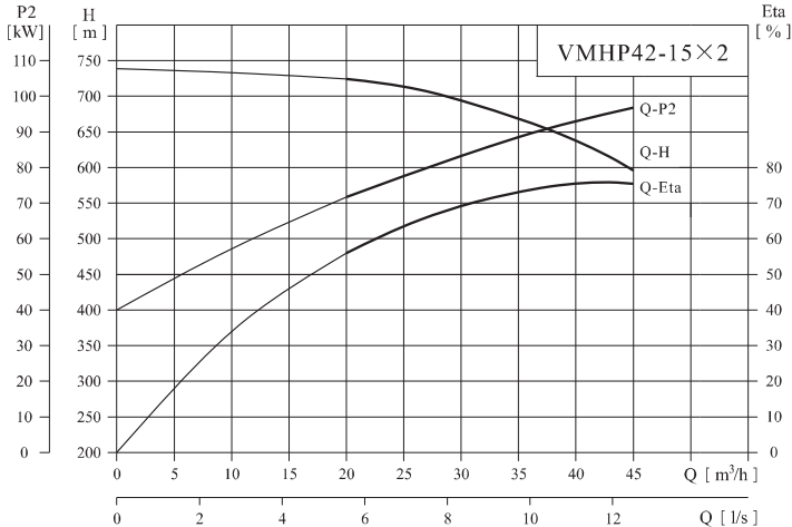
性能表VMHP42-15×2
