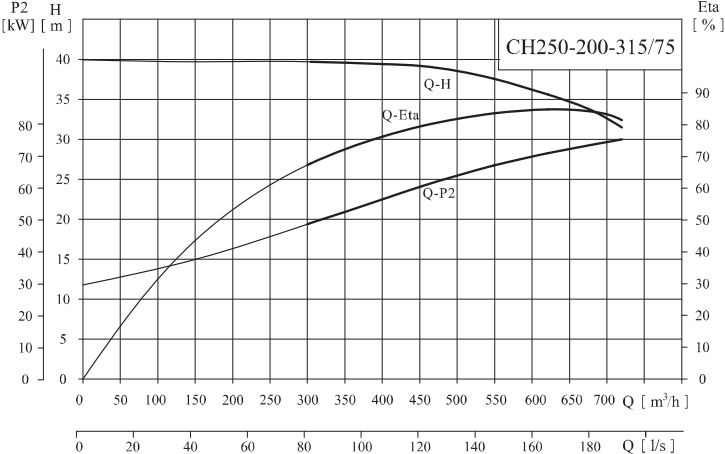
性能表CH250-200-315/75
