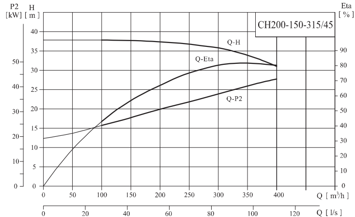
性能表CH200-150-315/45
