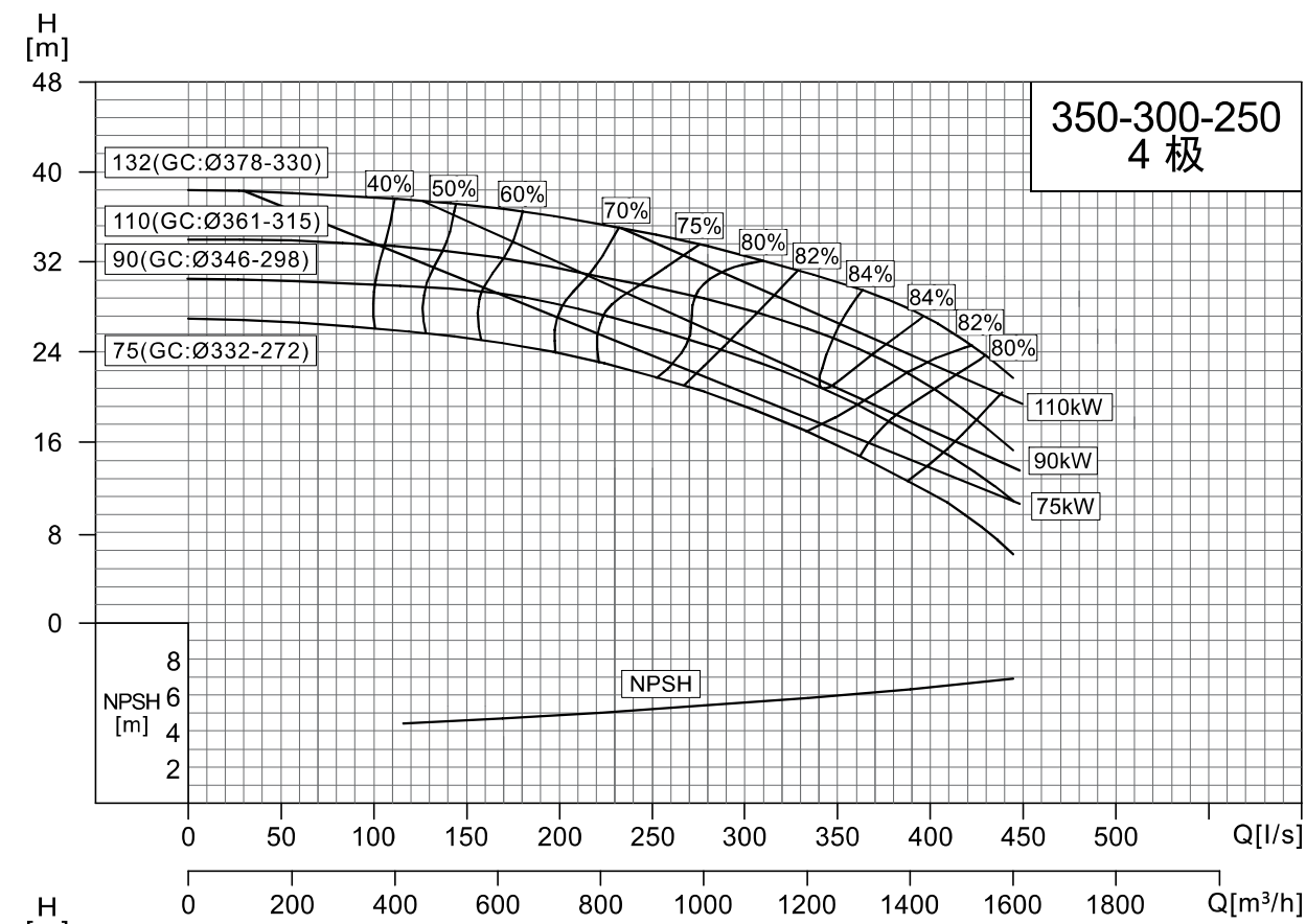
NISO,NIS,NISF350-300-250/350-300-315
