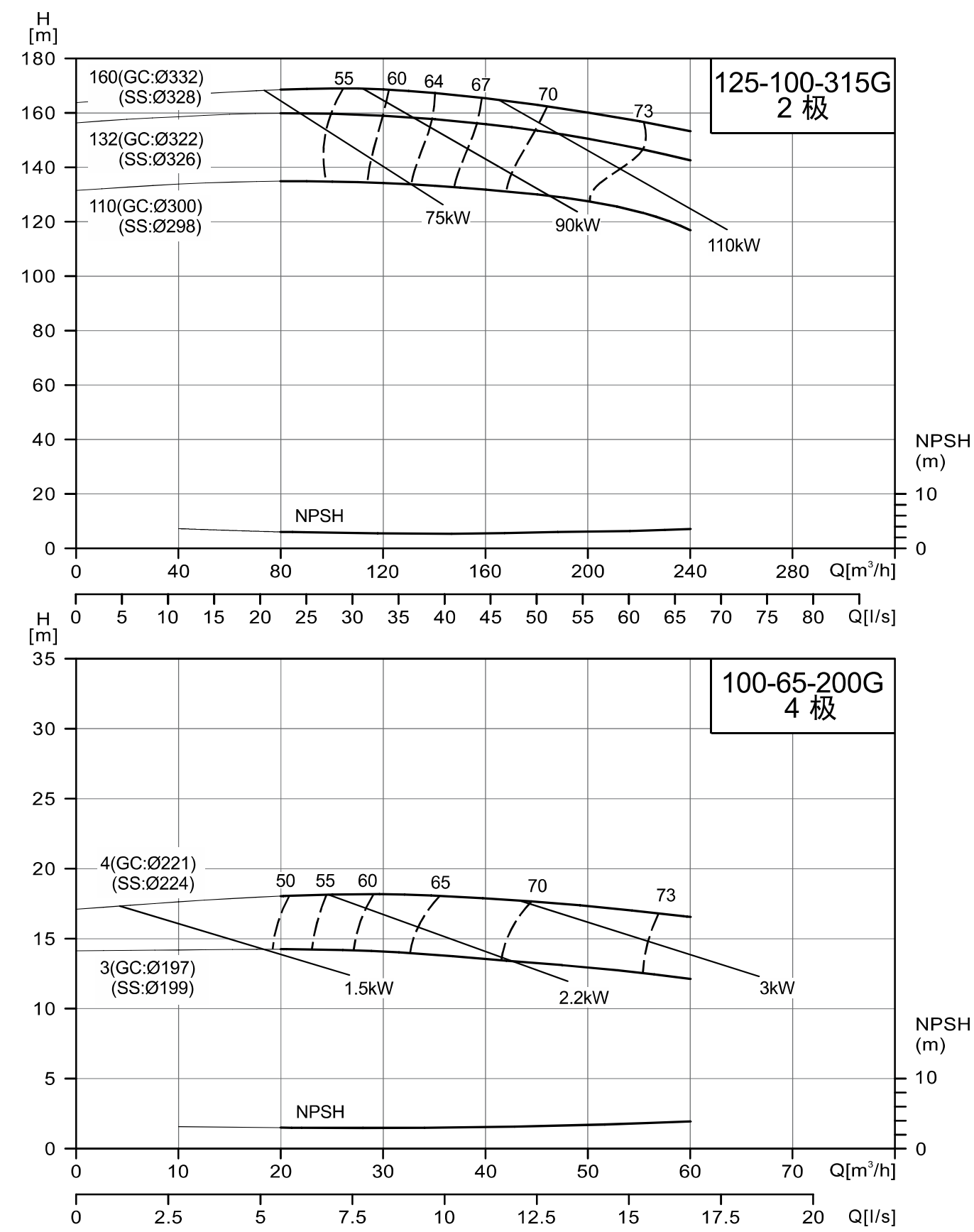
NISO/NIS/NISF125-100-315G/100-65-200G
