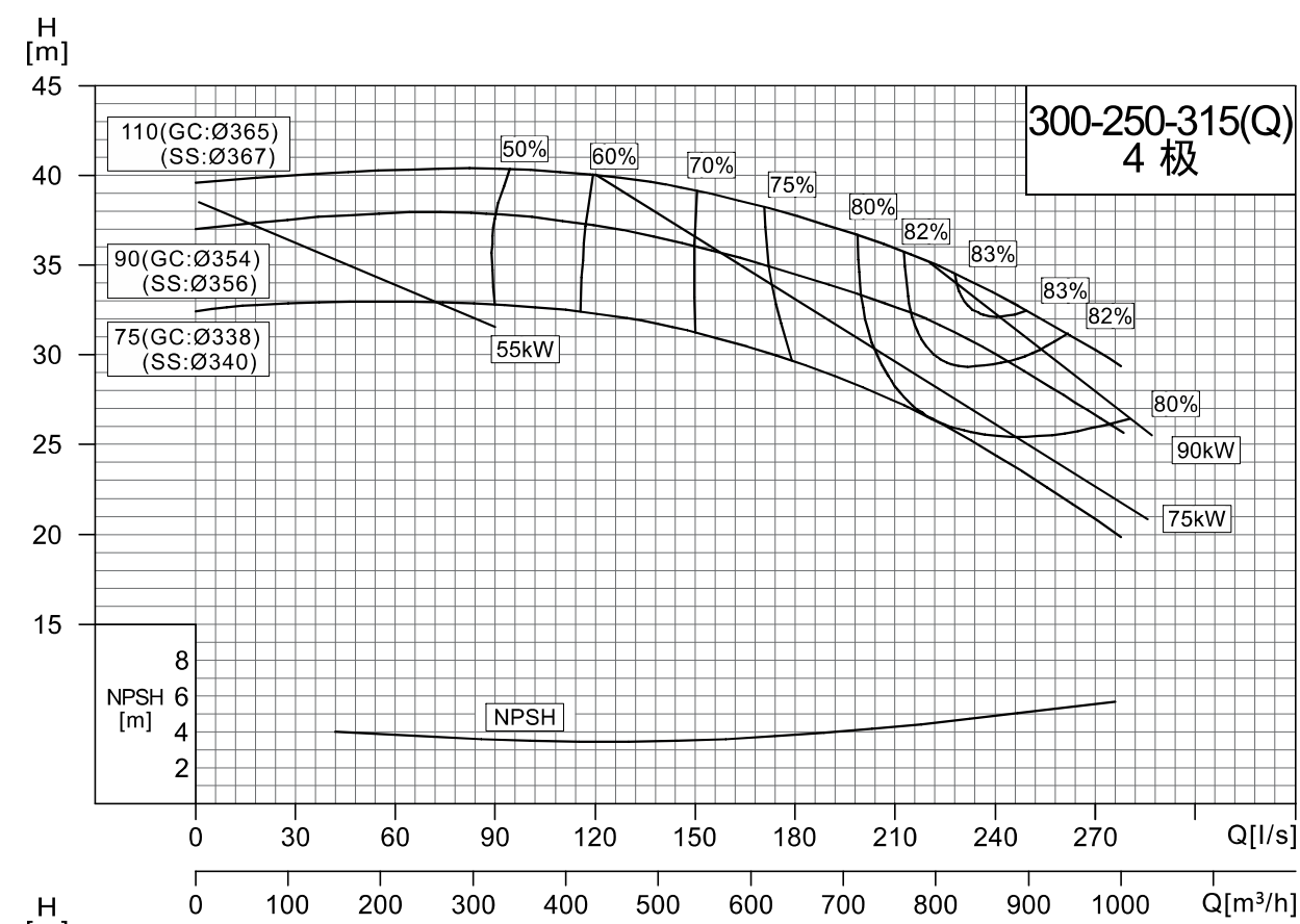
NISO,NIS,NISF300-250-315(Q)/300-250-315
