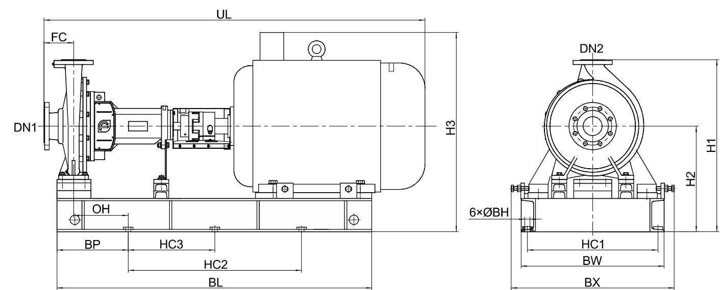
NISO*G,NISO*(Q)泵组外形尺寸图(槽钢底座结构)
