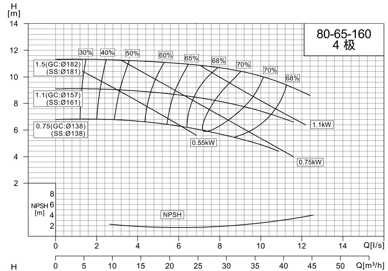
NISO,NIS,NISF80-65-160/100-65-200
