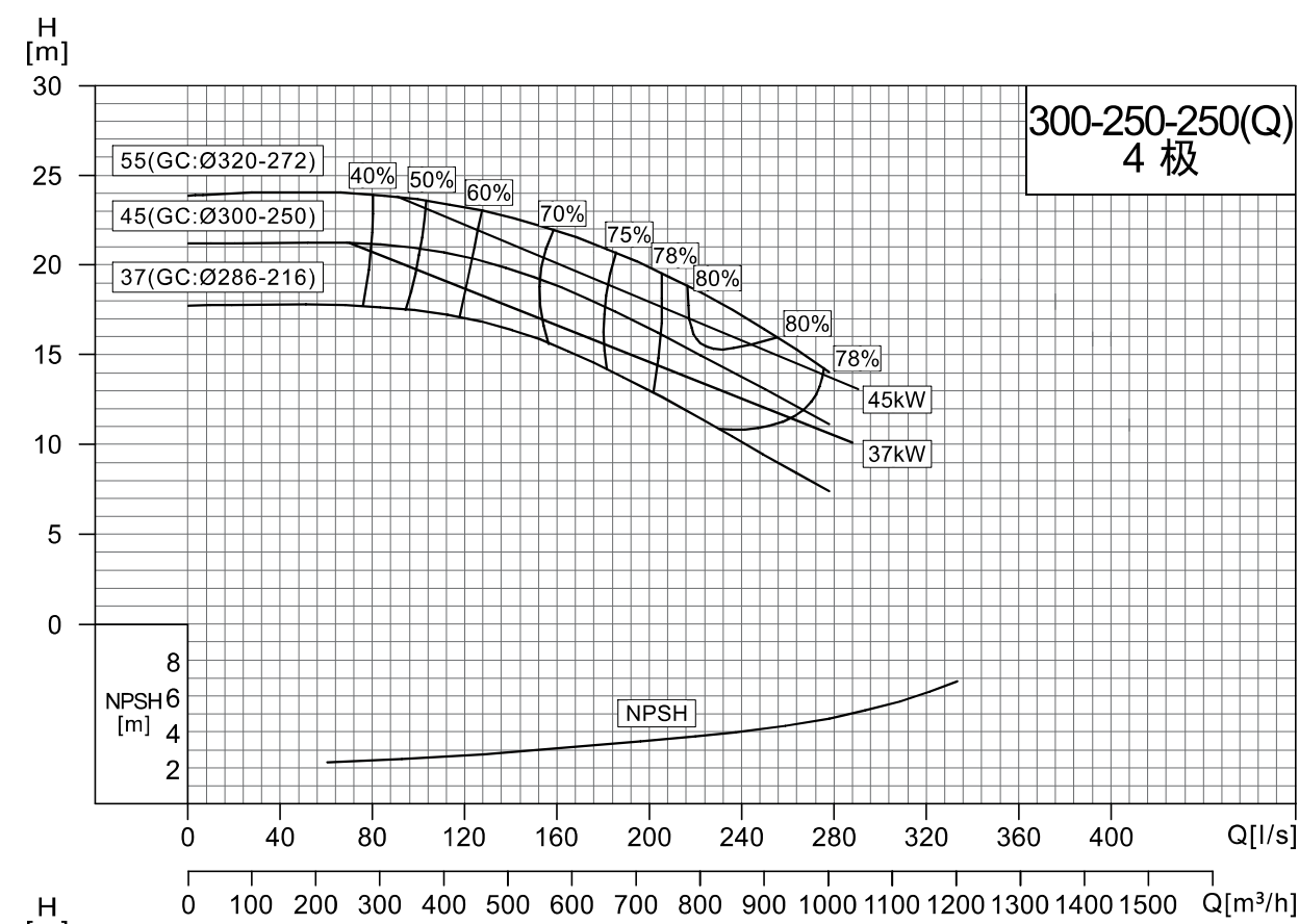
NISO,NIS,NISF300-250-250(Q)/300-250-250
