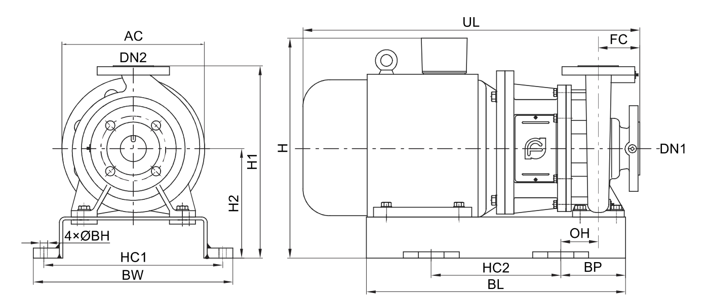
NIS,NISF泵外形尺寸图
