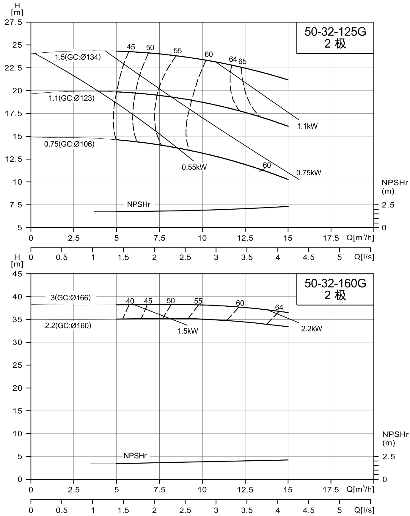
NISO/NIS/NISF50-32-125G/50-32-160G
