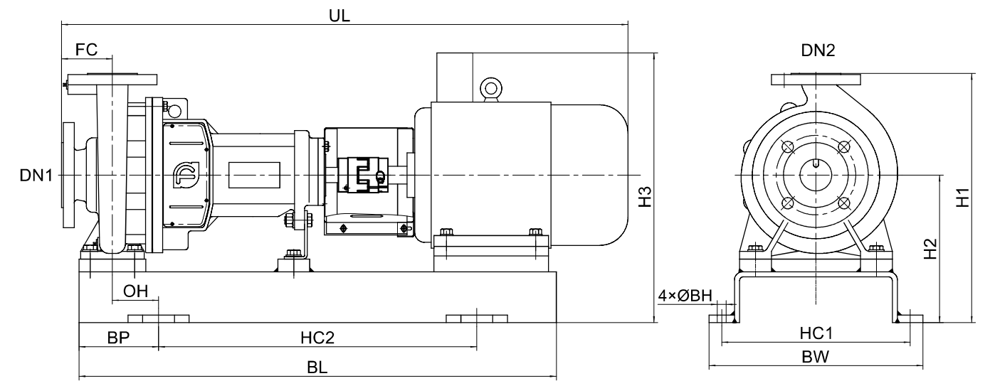
NISO*G,NISO*(Q)泵组外形尺寸表
