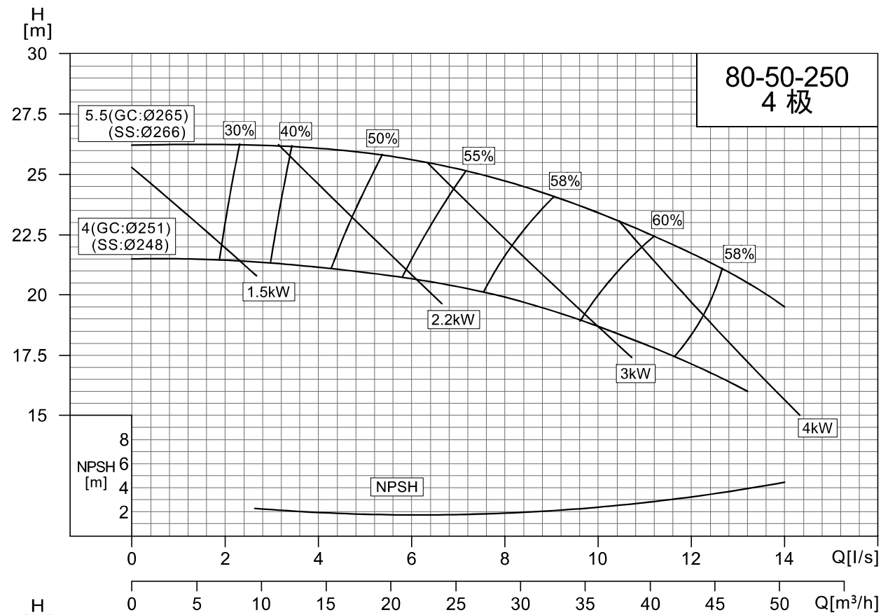
NISO,NIS,NISF80-50-250/80-50-315
