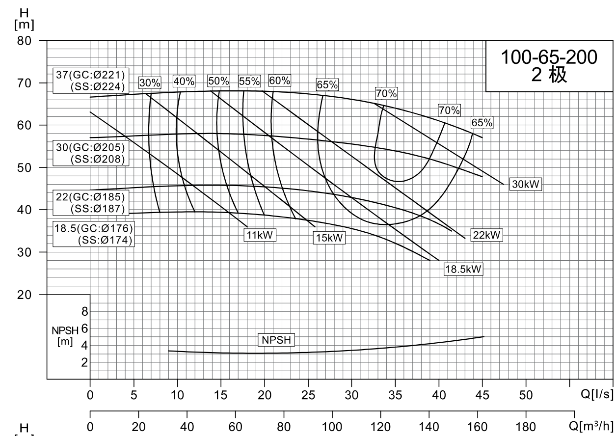
NISO,NIS,NISF100-65-200/100-65-250
