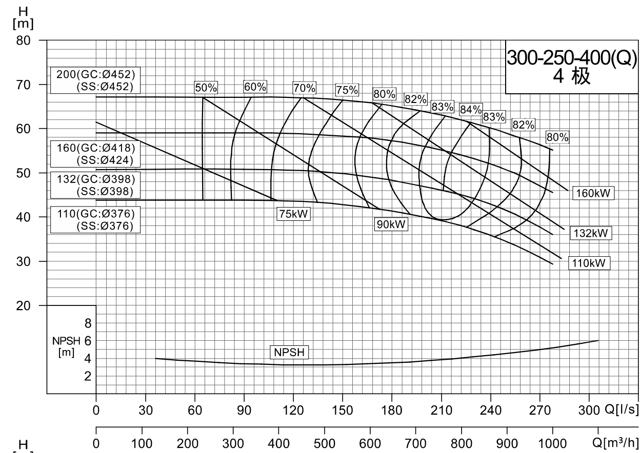
NISO,NIS,NISF300-250-400(Q)/300-250-400
