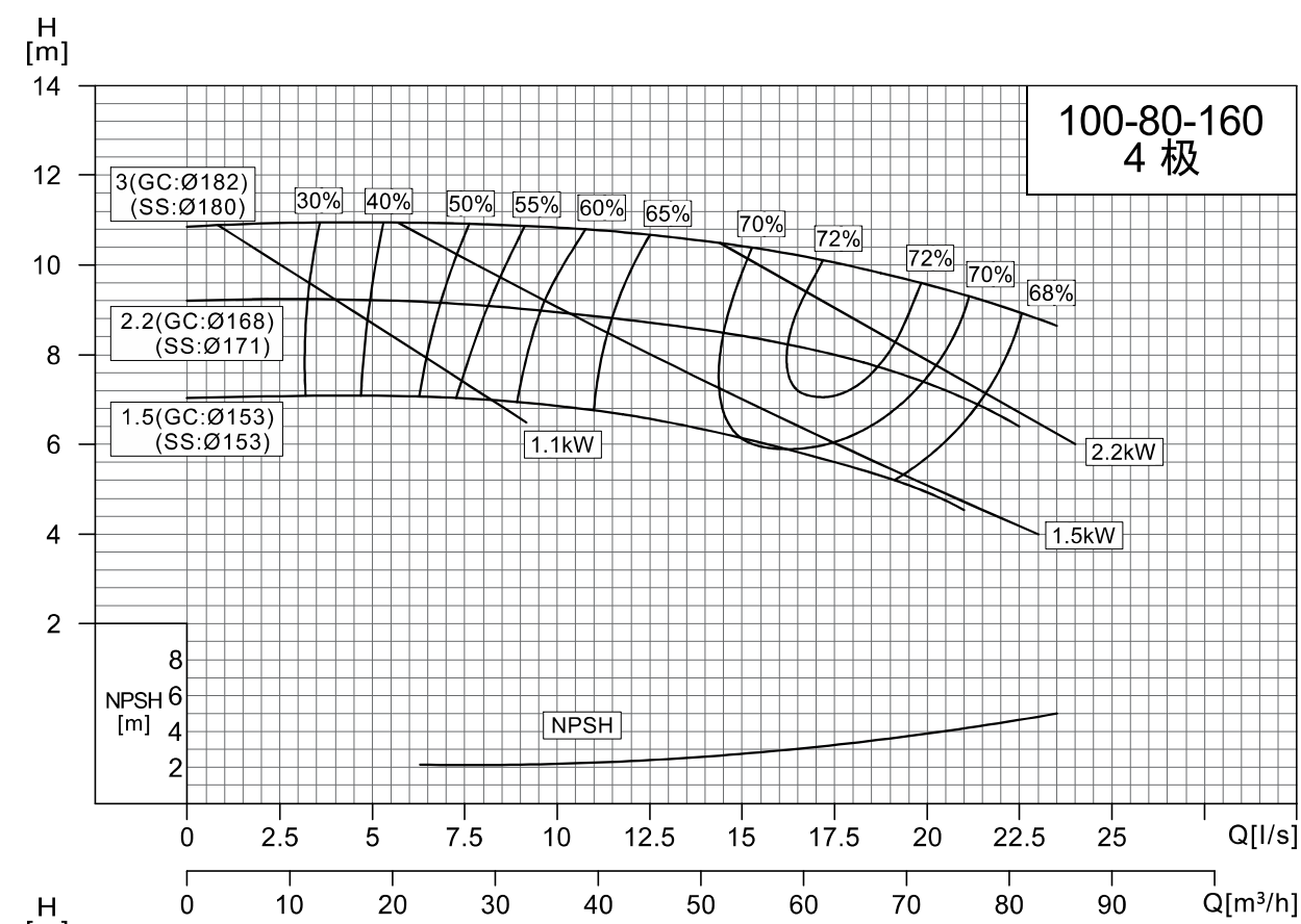
NISO,NIS,NISF100-80-160/125-100-200
