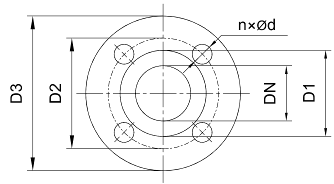
NIS/NISF*G,NIS/NISF*(Q)法兰
