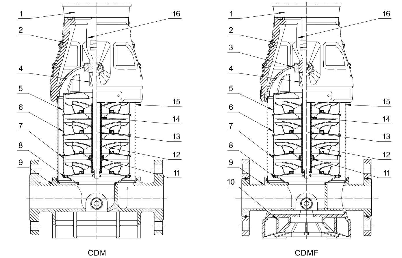
CDM10,15,20 材料表
