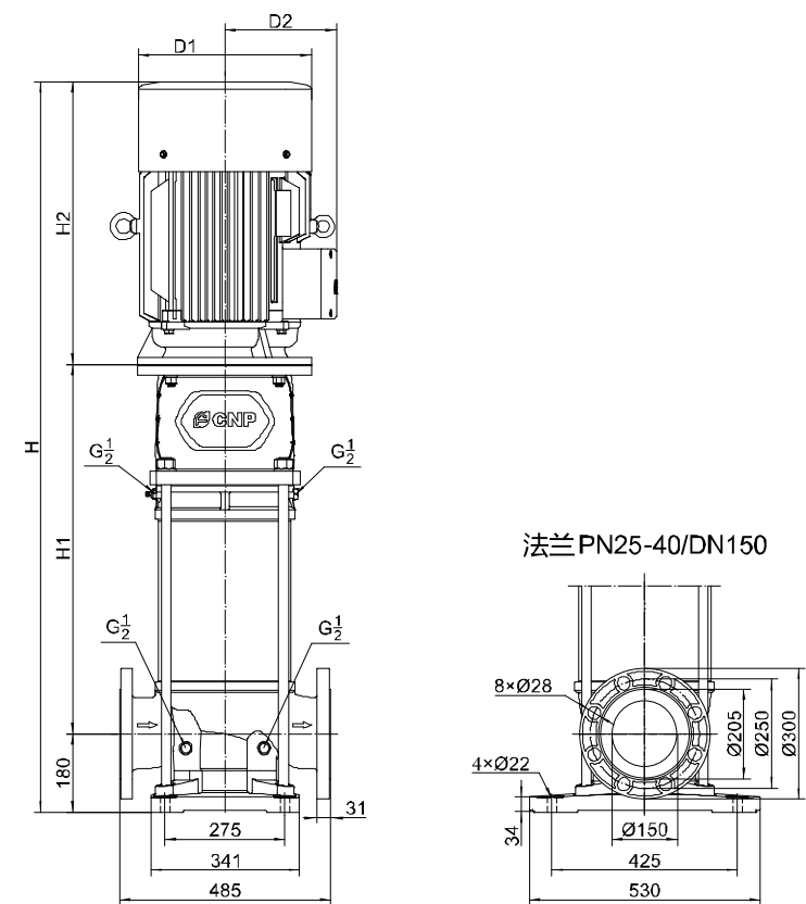
CDM/CDMF125安装尺寸图
