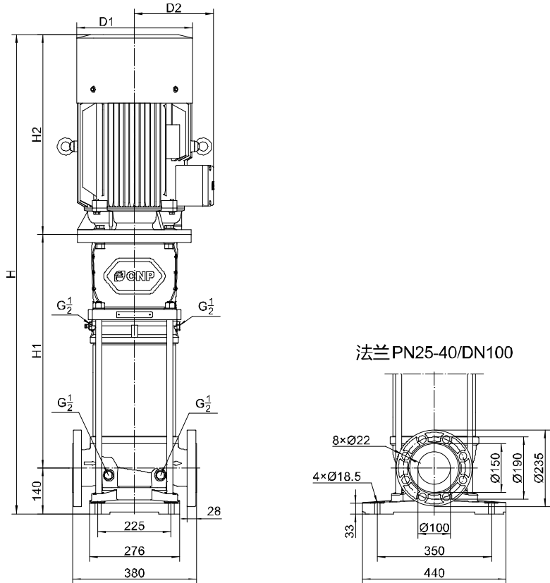
CDM/CDMF95安装尺寸图
