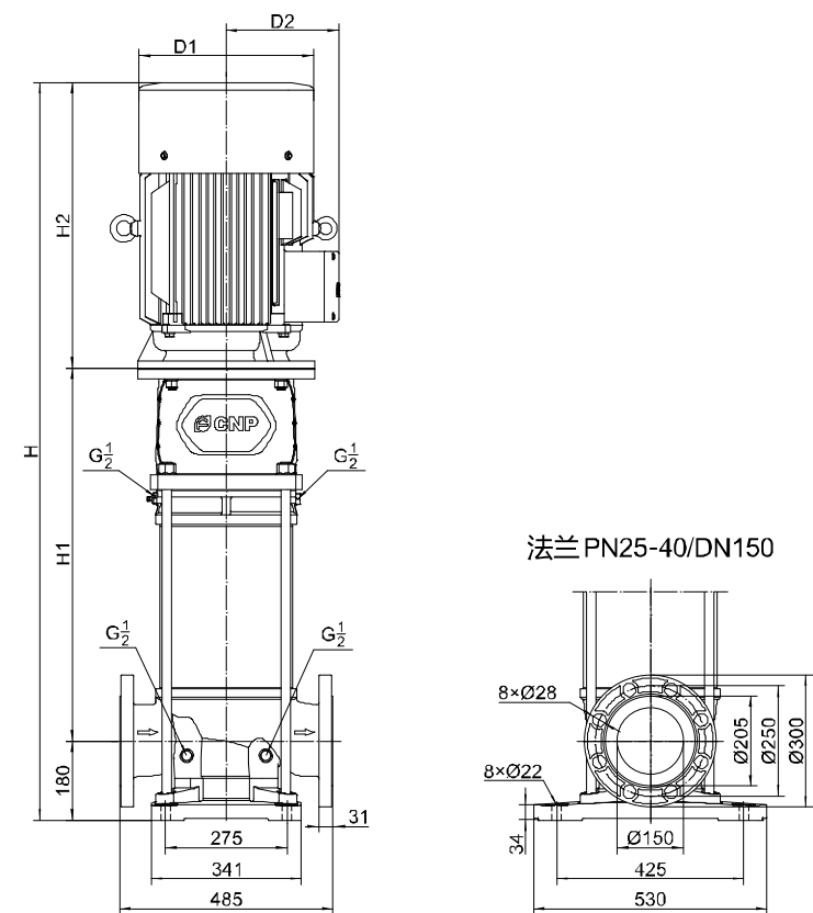
CDM/CDMF155安装尺寸图
