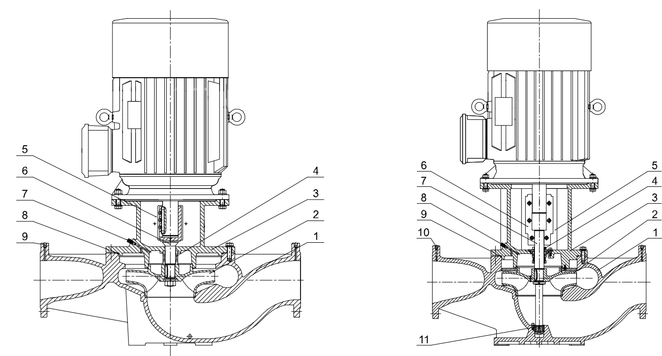
截面图TD32-TD150、TD200(≤18.5kW) 截面图TD200-TD250便拆式 加长轴
