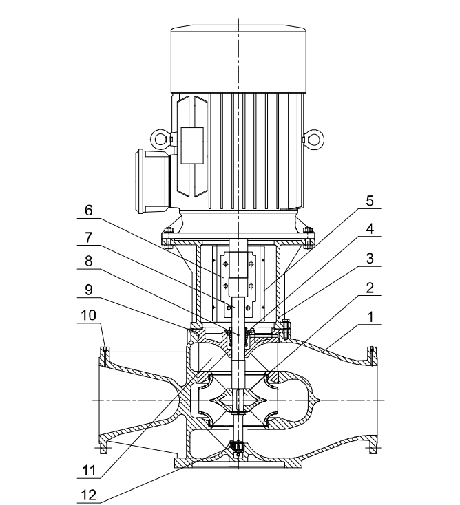
TD300材料表
