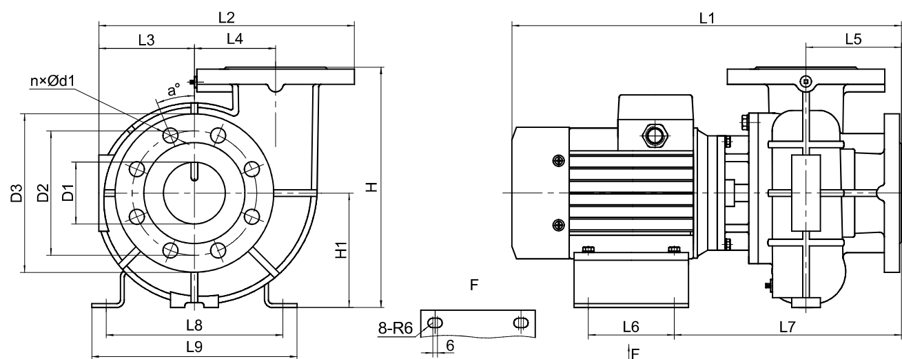
WLT/WLTS/WLTSF(50Hz)安装尺寸图
