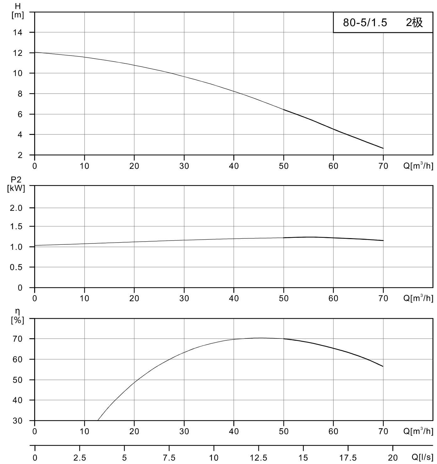
WLT/WLTS/WLTSF(50Hz)性能曲线
