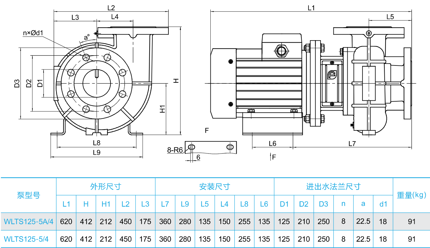
WLTS(60Hz)安装尺寸图
