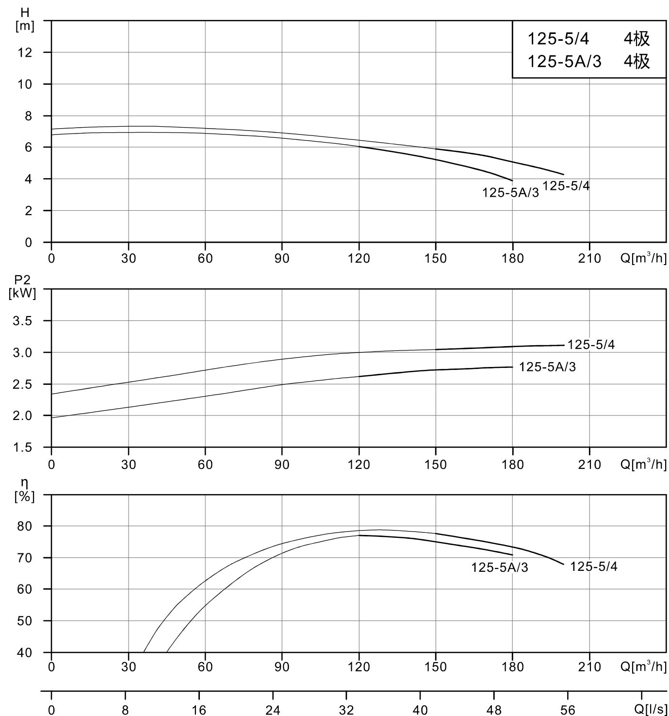
WLT/WLTS/WLTSF(50Hz)性能表
