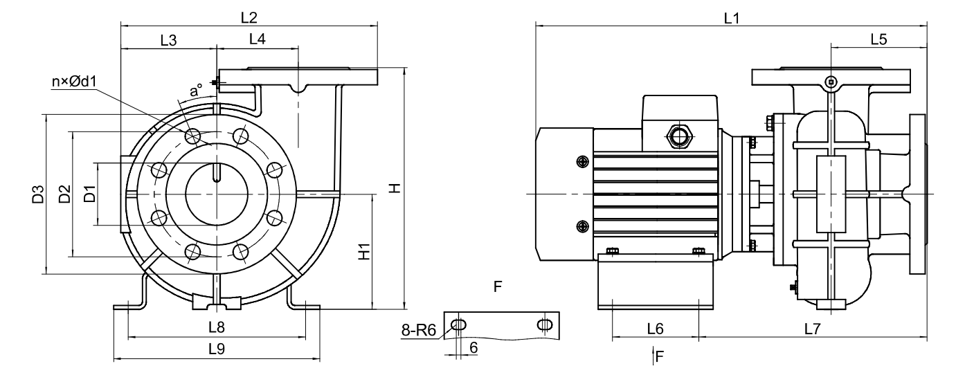
WLT/WLTS/WLTSF(50Hz)安装尺寸图
