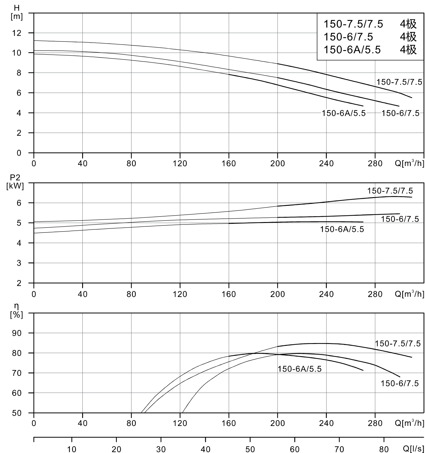
WLT/WLTS/WLTSF(50Hz)性能表
