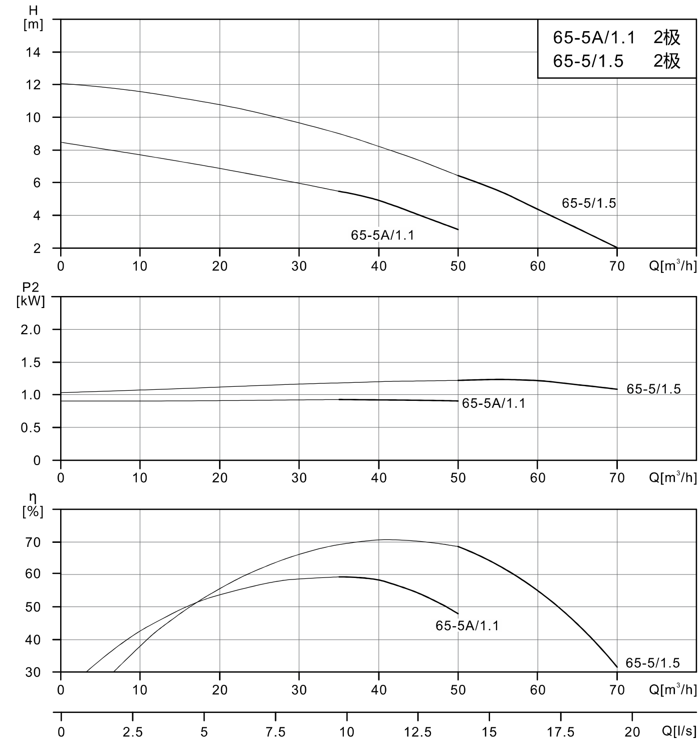
WLTS(60Hz)性能曲线
