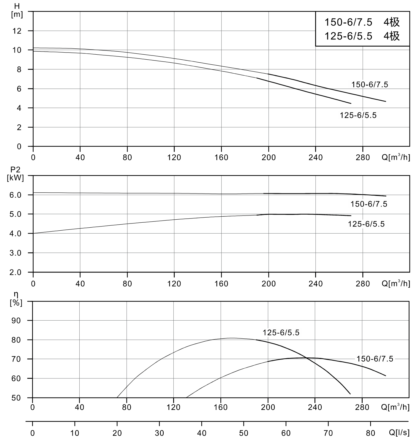
WLTS(60Hz)性能曲线
