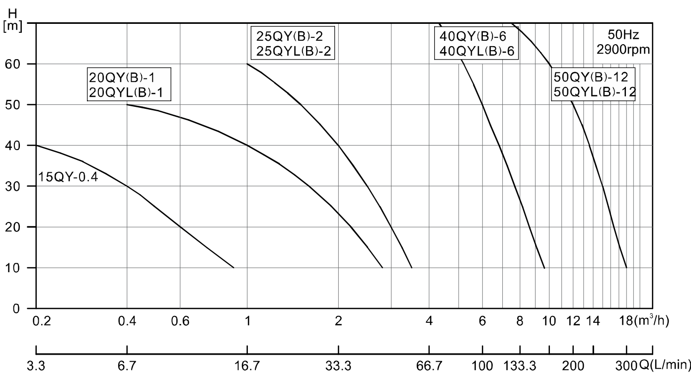
性能曲线
