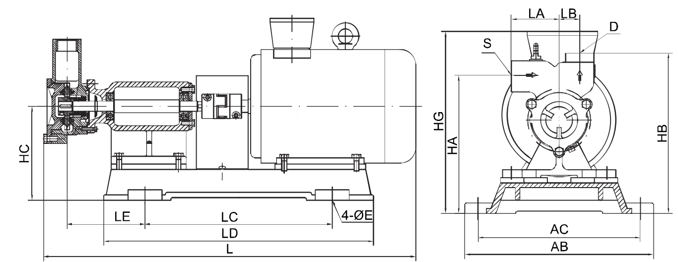
QYL(B)安装图
