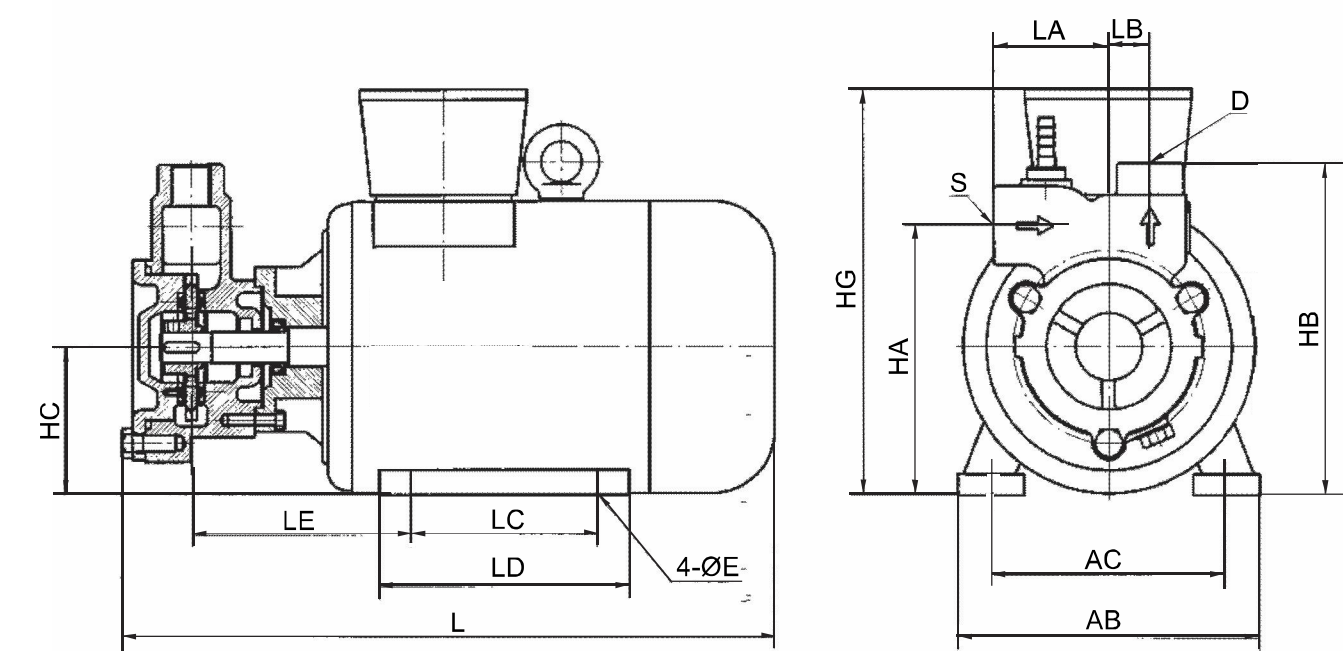
QY(B)安装图
