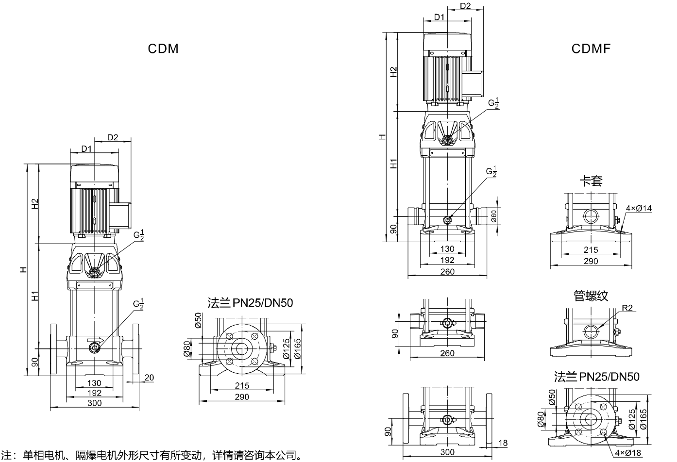
CDM/CDMF15安装尺寸图
