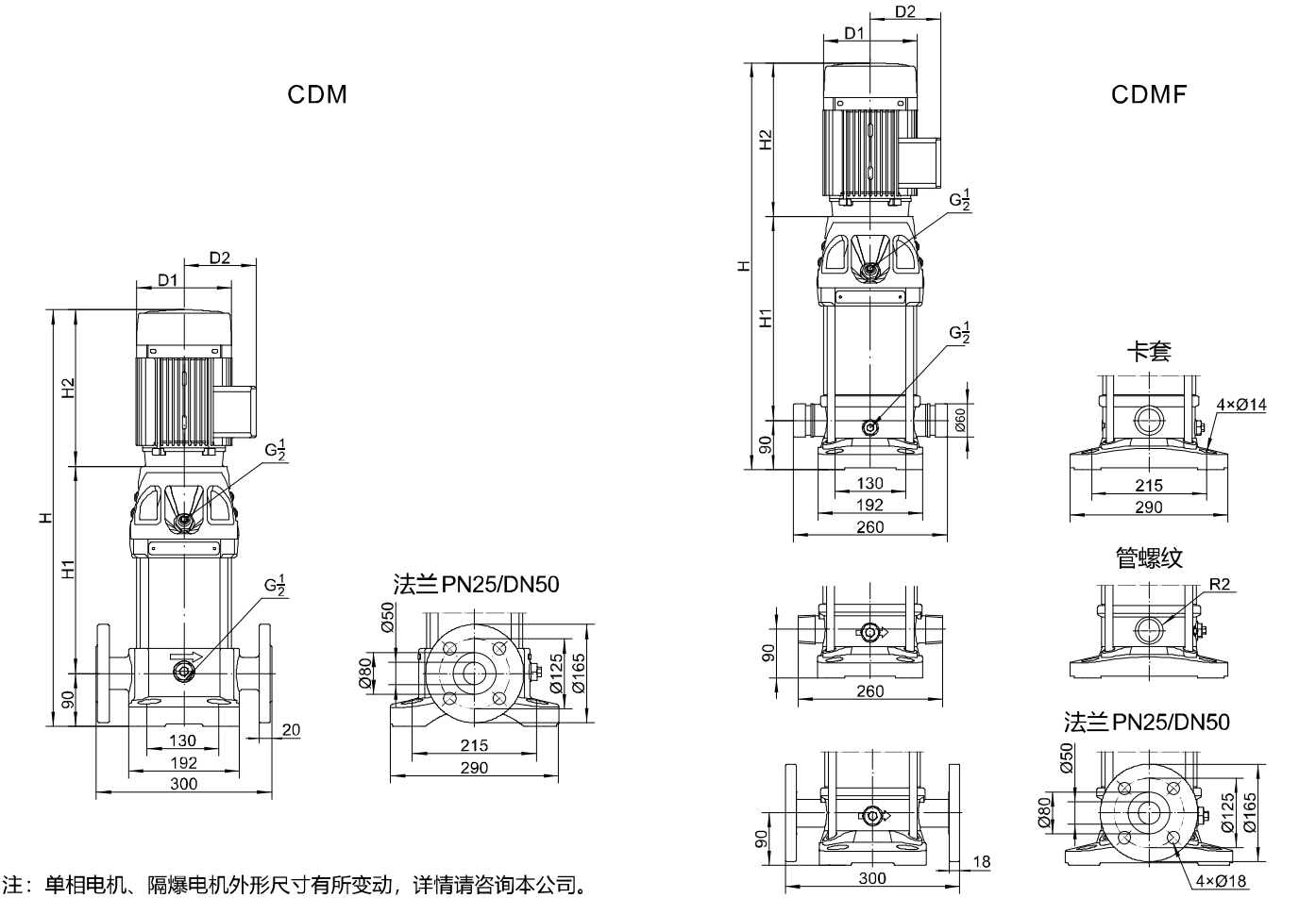
CDM/CDMF20安装尺寸图
