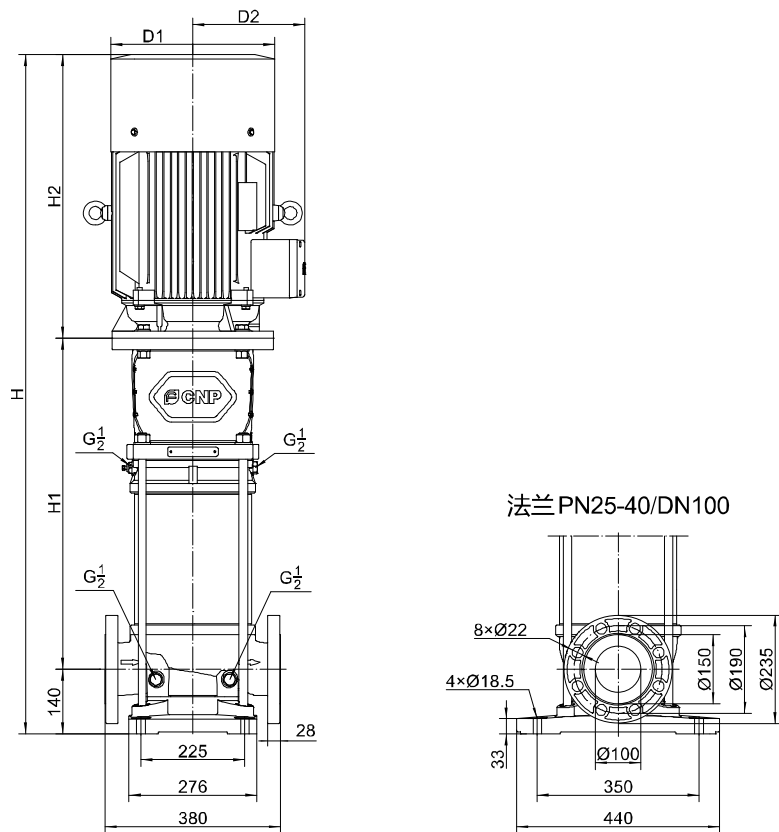
CDM/CDMF95安装尺寸图
